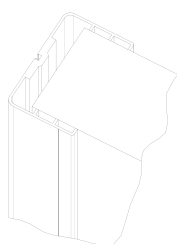
PD-3, 4 og 5 Aluminiumskarm Fast karm for veggykkelser PD-3: 75 mm PD-4: 80 mm PD-5: 100 mm
